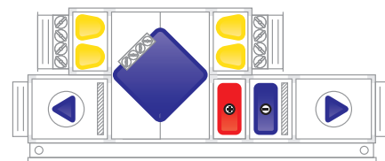
Пластиновый рекуператор
