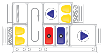
Роторный рекуператор
