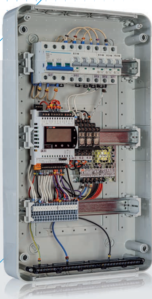
Вид шкафа без крышки
