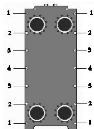
Рис. 10. Разборка теплообменника
