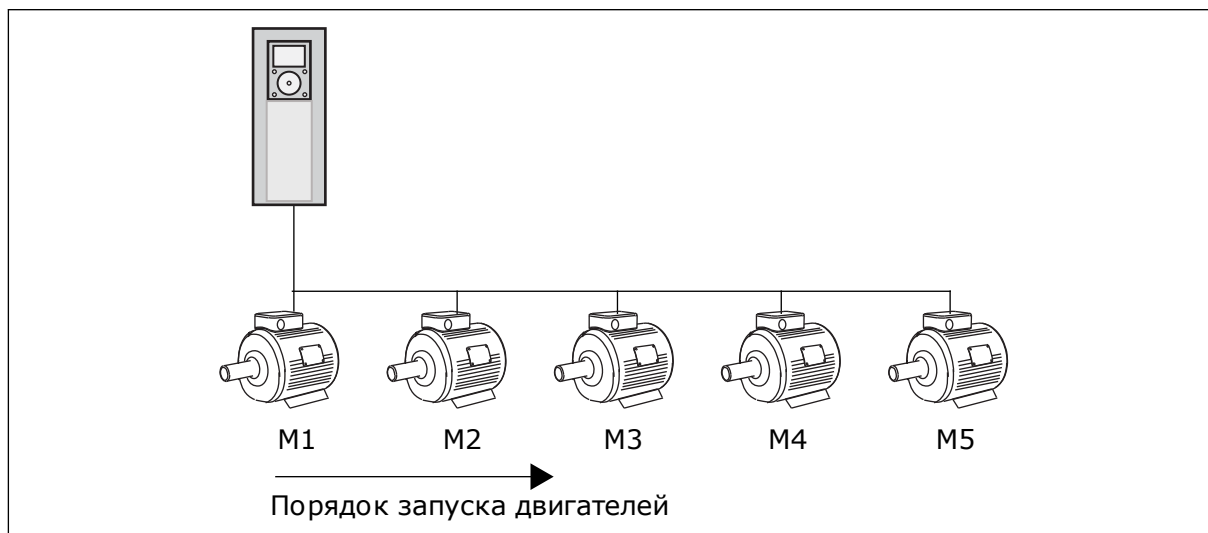
Рис. 80: Логика блокировки 1
