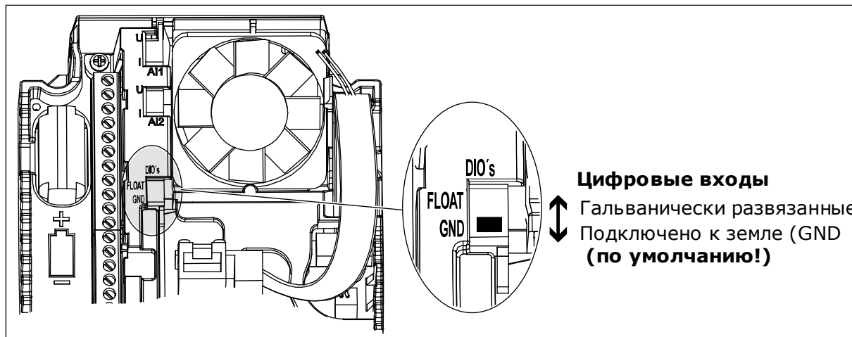
Рис. 9: DIP-переключатель
