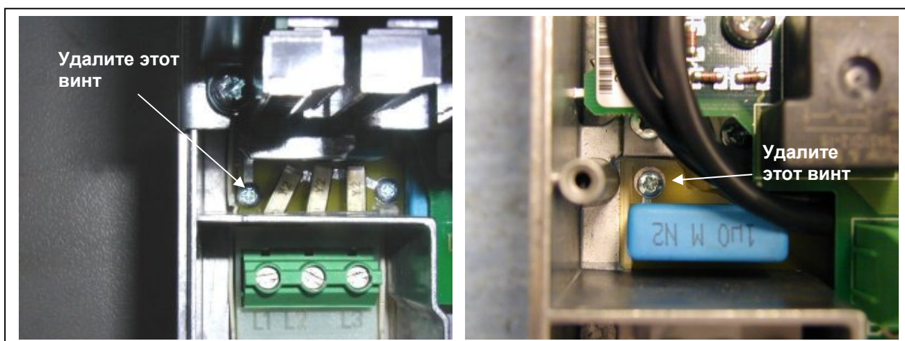
Рисунок 6-2. Изменение класса защиты по ЭМС, FR4 (слева) и FR5 (справа)
