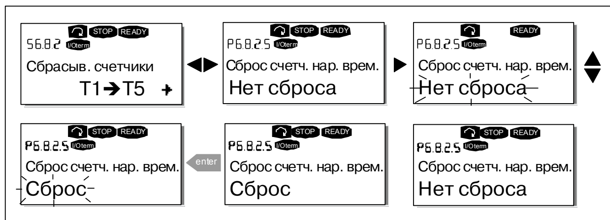
Рисунок 7-24. Сброс счетчиков
