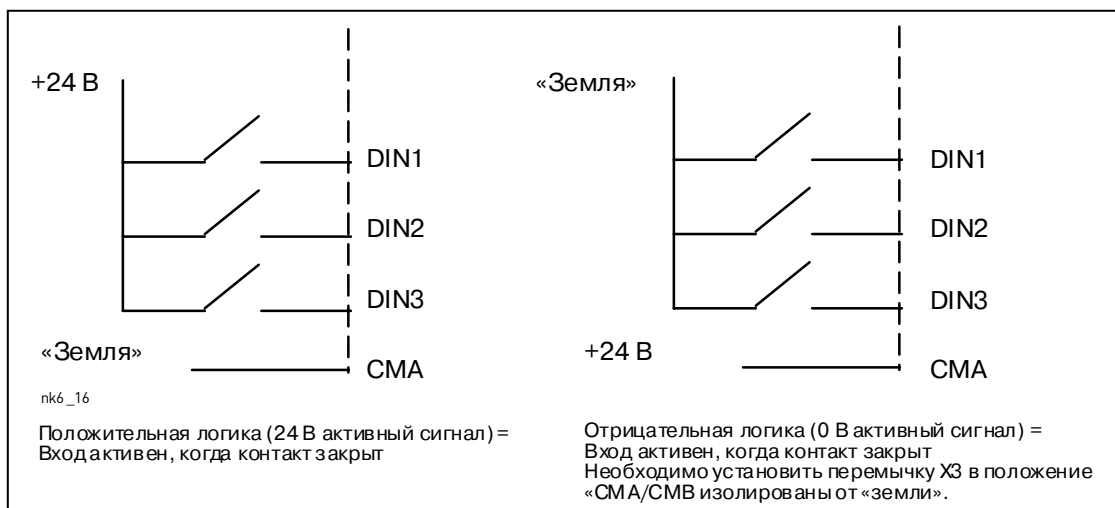
Рисунок 6-27. Положительная/отрицательная логика
