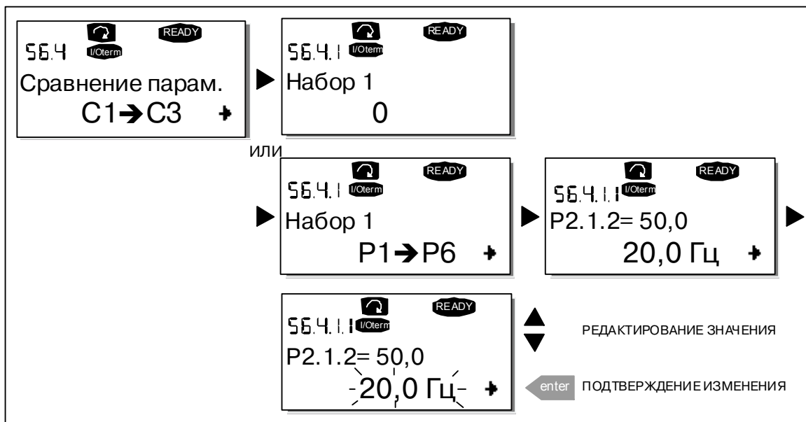
Рисунок 7-13. Сравнение параметров
