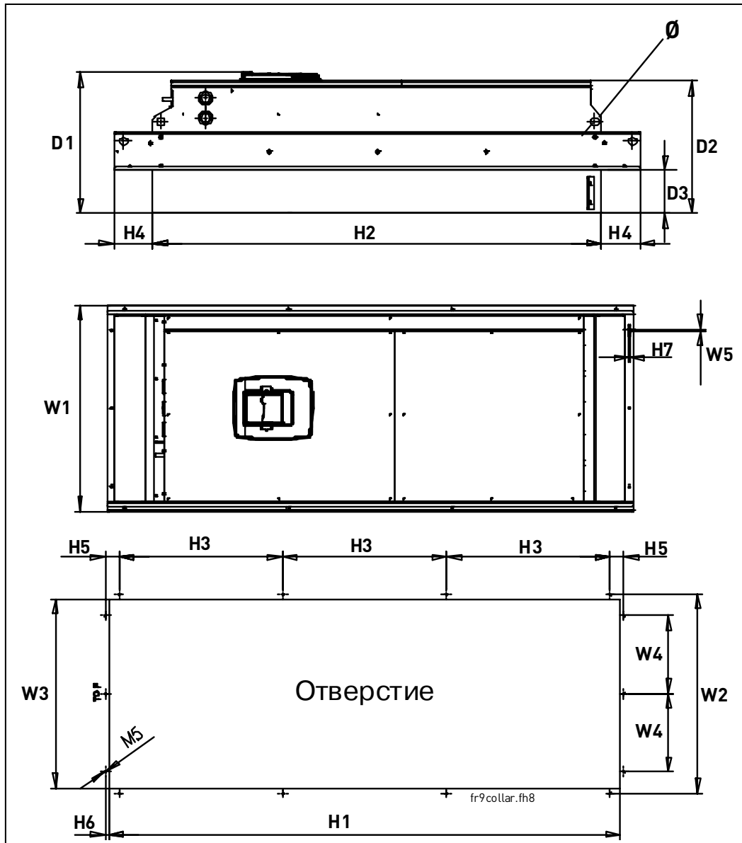
Рисунок 5-8. Габариты преобразователей частоты Vacon NX фланцевого исполнения, типоразмер FR9
