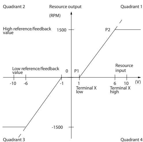
Рисунок 3.16 Зона нечувствительности
