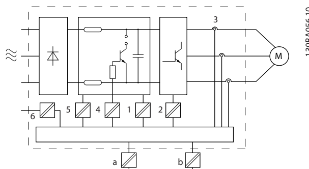
Рисунок 3.27 Гальваническая развязка
