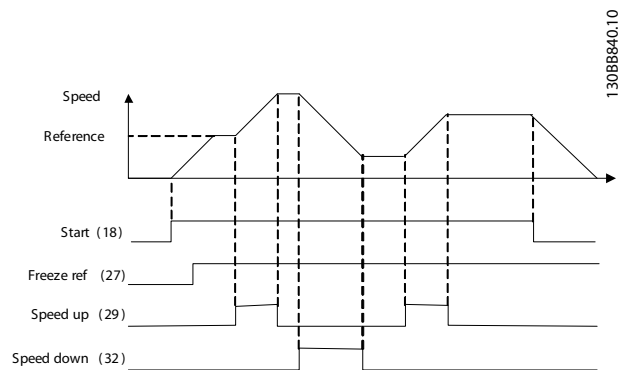
Рисунок 8.3 Увеличение/снижение скорости
