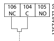
Рисунок 7.54 Межкомпонентные соединения термореле тормозного резистора
