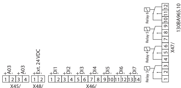
Рисунок 9.17 Электрические подключения MCB 113
