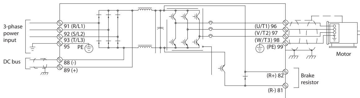
Рисунок 3.1 Принцип управления
