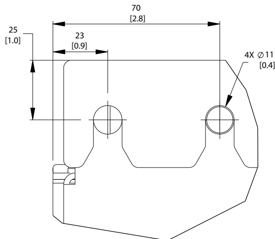
Рисунок 6.22 Детальный чертеж верхнего монтажного отверстия, D8h
