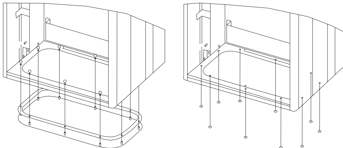
Рисунок 4.25: Монтаж нижней платы, E7
