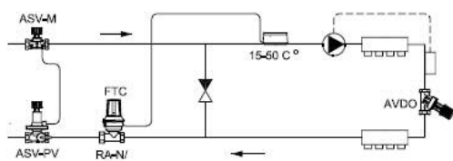
Система обогрева полов
