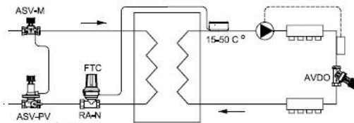
Радиаторная система отопления или обогрева пола с теплообменником
