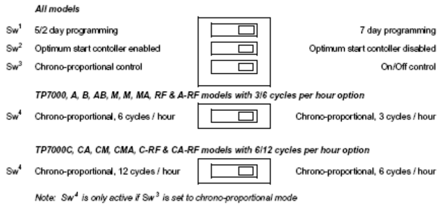
Рис. 10. Назначение переключателей
