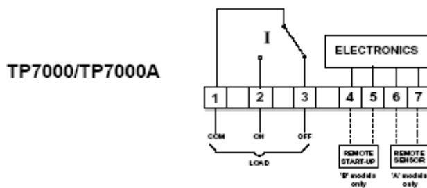
Рис.11. Электрическая схема подключения
