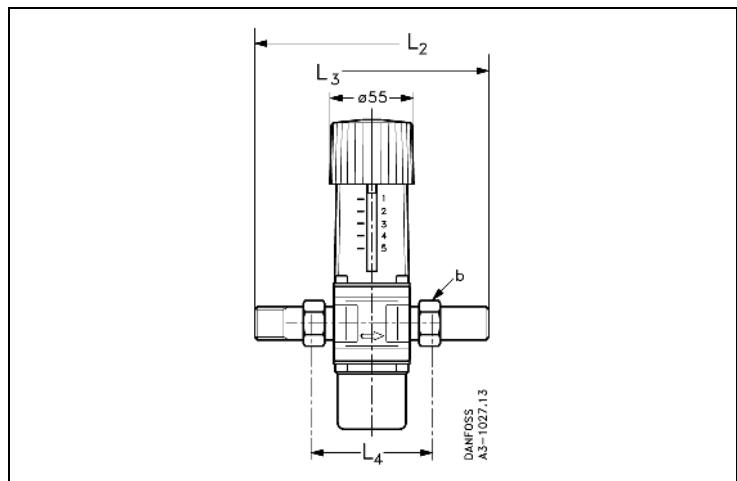
Рис. 5. Габаритные и присоединительные размеры клапана-ограничителя температуры FJV (с наружной резьбой).
