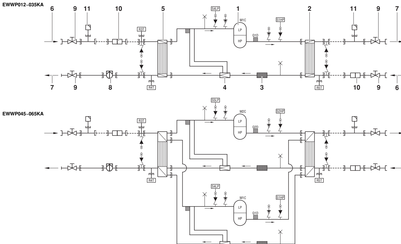
Рисунок: Функциональная схема чиллера
