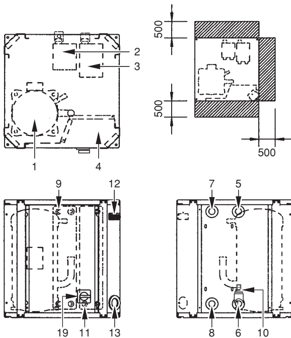
Рисунок: Основные элементы
