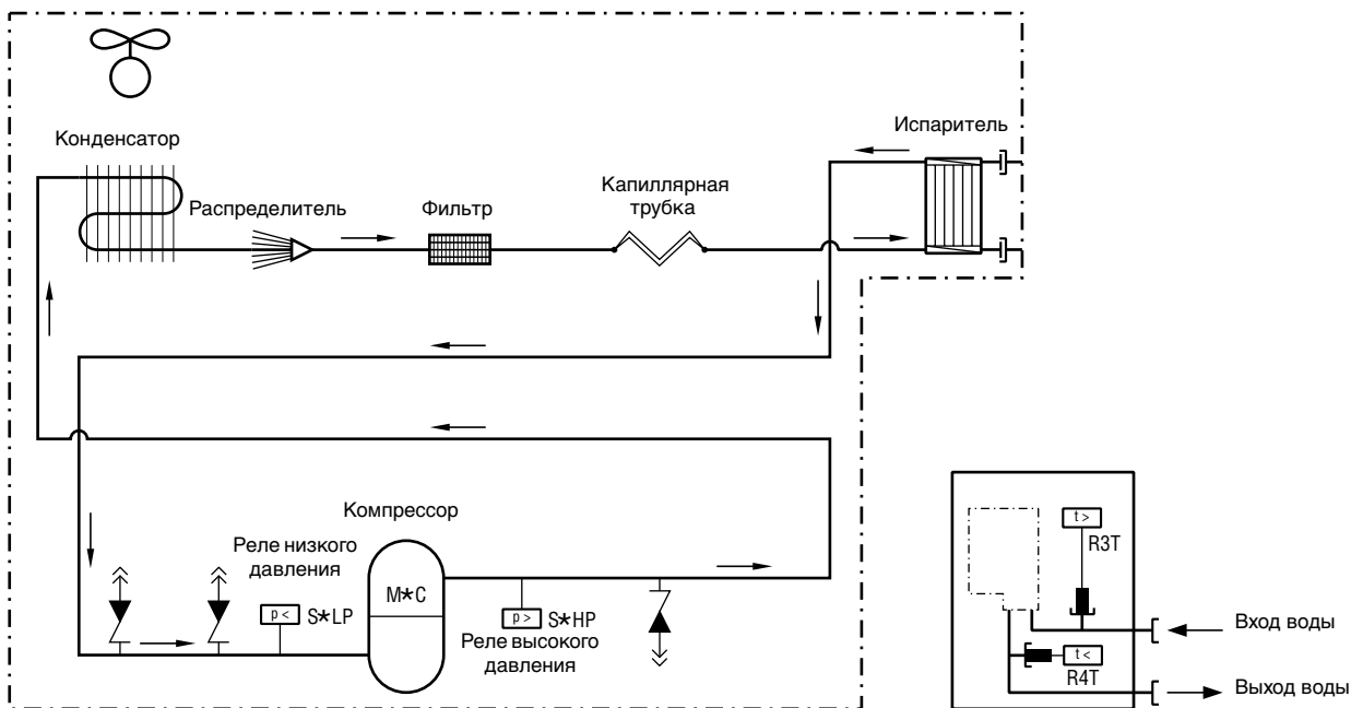
Рисунок - Функциональная схема чиллера
