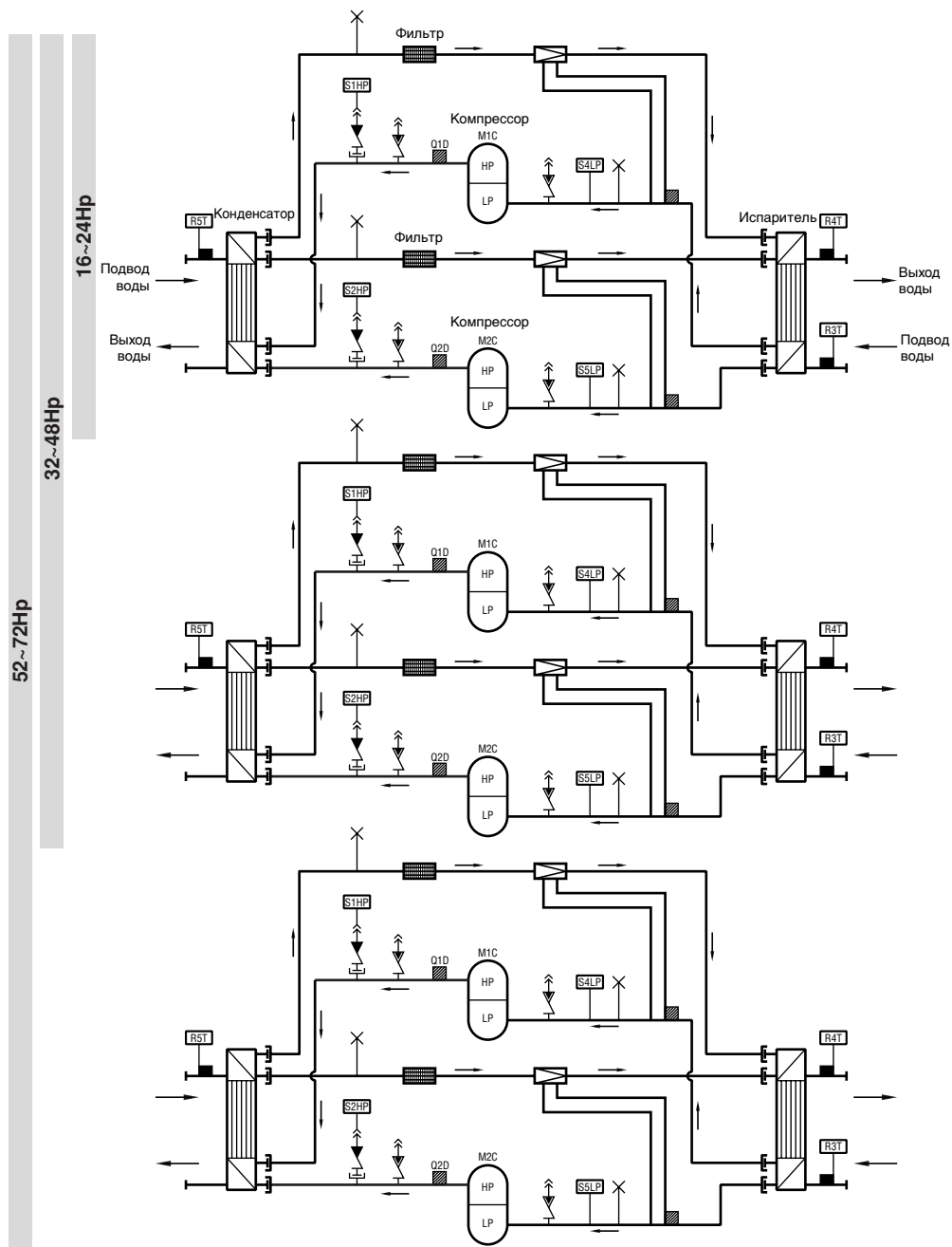
Рисунок - Функциональная схема чиллера
