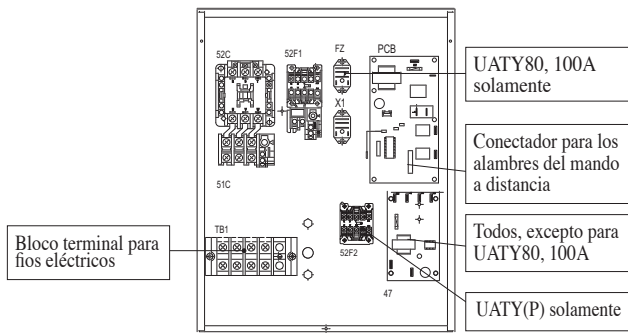
MÓDULO DE CONTROL UAT(Y)80, 100A, UAT(Y)(P)120A
