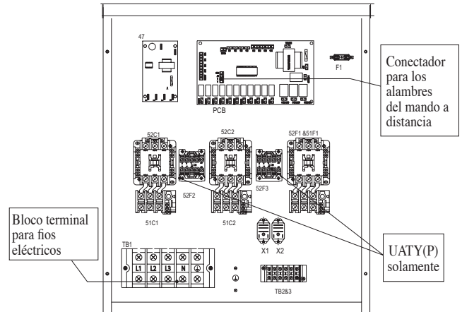
MÓDULO DE CONTROL UAT(Y)(P)360, 420A
