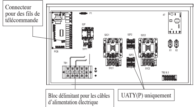
MODULE DE COMMANDE UAT(Y)(P)360, 420A
