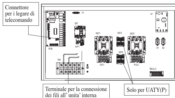
MODULO DI CONTROLLO UAT(Y)(P)360, 420A
