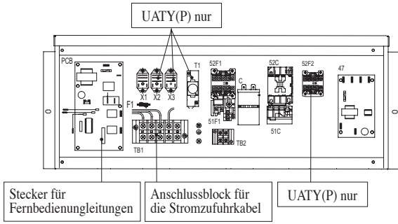
STEUERMODUL UAT(Y)(P)60A
