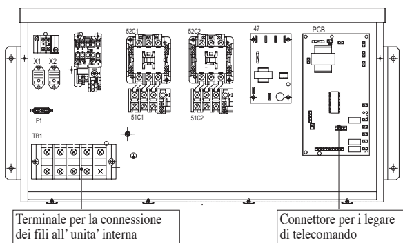
MODULO DI CONTROLLO UAT(Y)(P)250A
