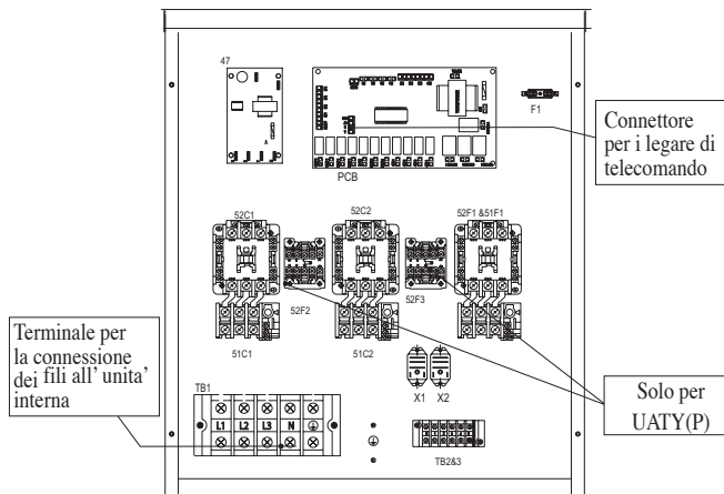
MODULO DI CONTROLLO UAT(Y)(P)360, 420A
