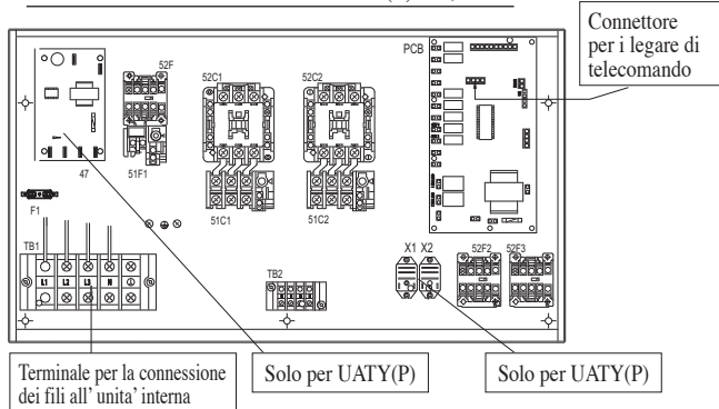
MODULO DI CONTROLLO UATY(P)150, 200A
