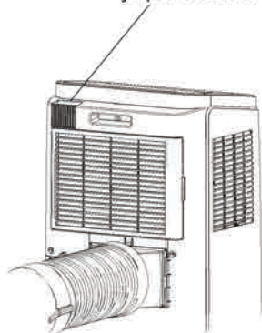
Крюк для фиксации пульта дистанционного управления
