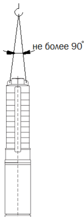
Рисунок 4 Схема строповки агрегата электронасосного
