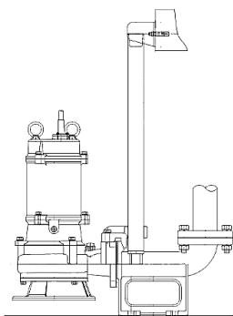
Исполнение с автоматической трубной муфтой (АС+артикул
