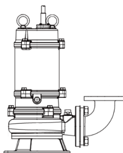
Исполнение с коленом под фланец (ЕF+артикул аксессуара)
