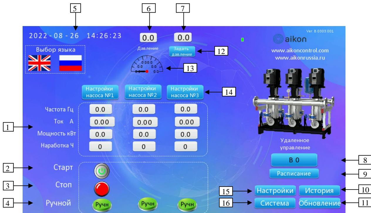
Рисунок 2. Главный экран панели управления с программой для трех насосов.
