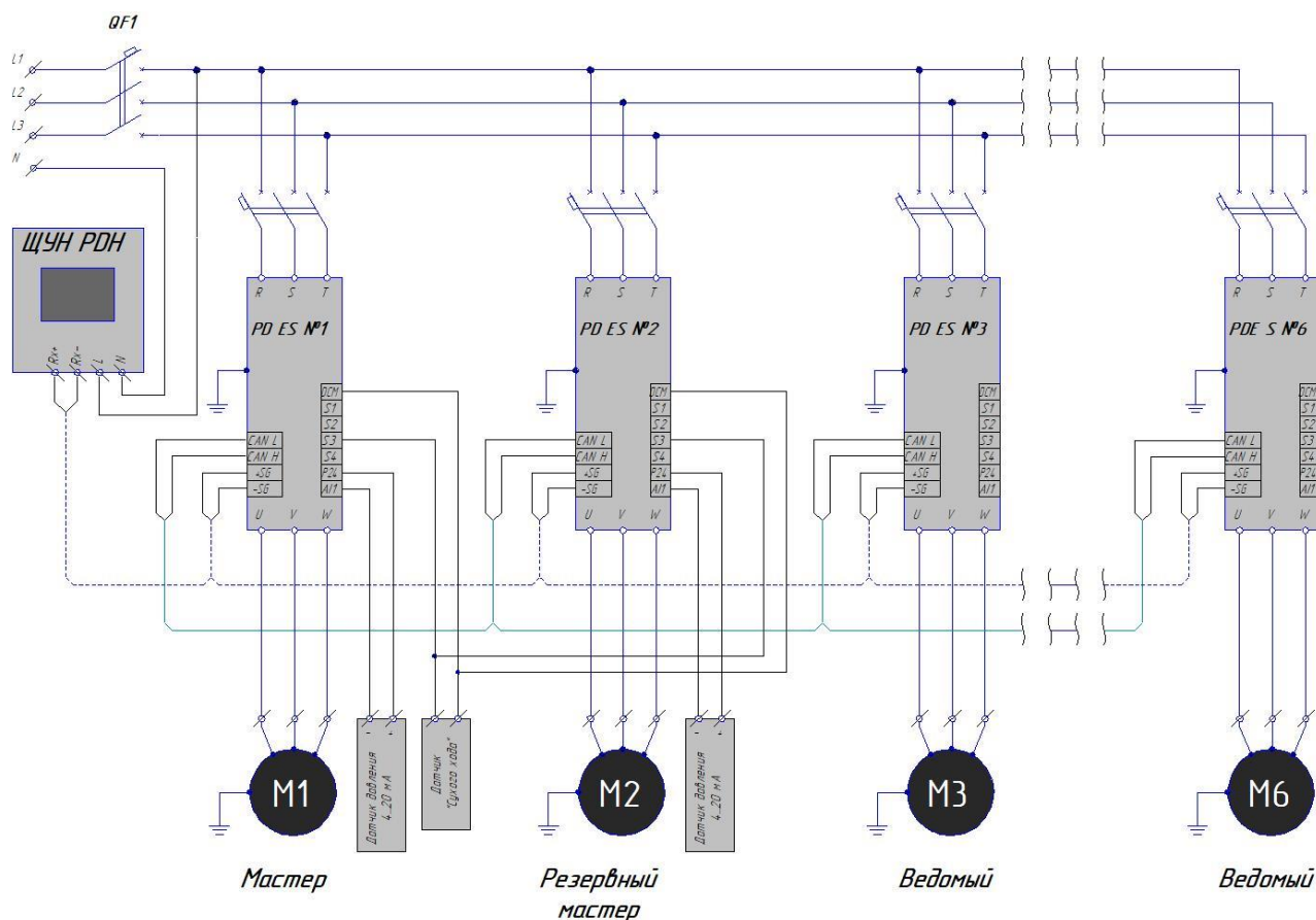
Рисунок 1. Структурная схема подключения ЩУН PD Н к контроллерам с функцией преобразования частоты PDES на насосной станции.
