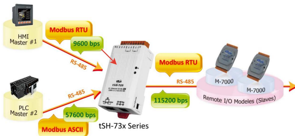
Рисунок 9. Схема организации сети с двумя мастерами.
