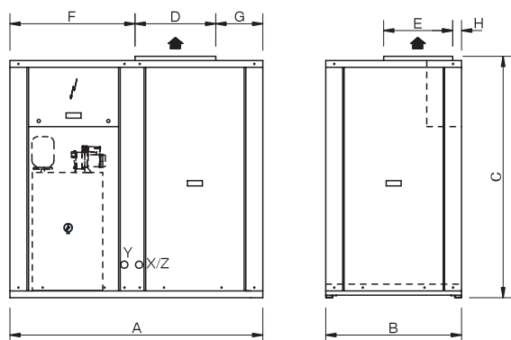
Вид "А-А"
