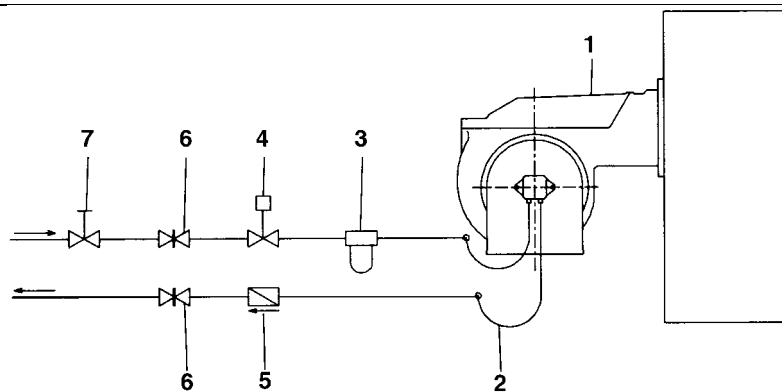
Рис. 3 - Двухтрубная система
