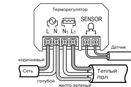
Подключение к 2-х проводной линии
