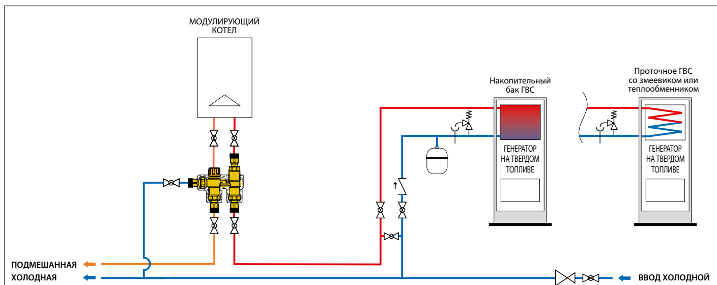
Прикладная схема комплекта SOLARINCAL-T PLUS серии 263 с генератором на твердом топливе
