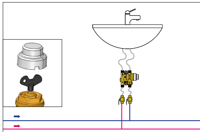
Прикладная схема термостатического смесителя кода 521201
