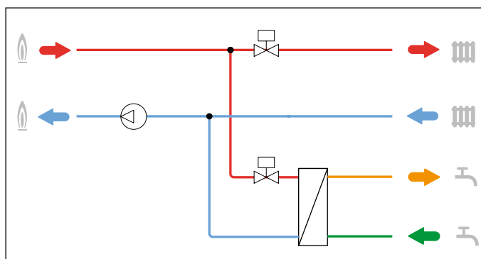
Схема гидравлической обвязки SATK204/SATK224
