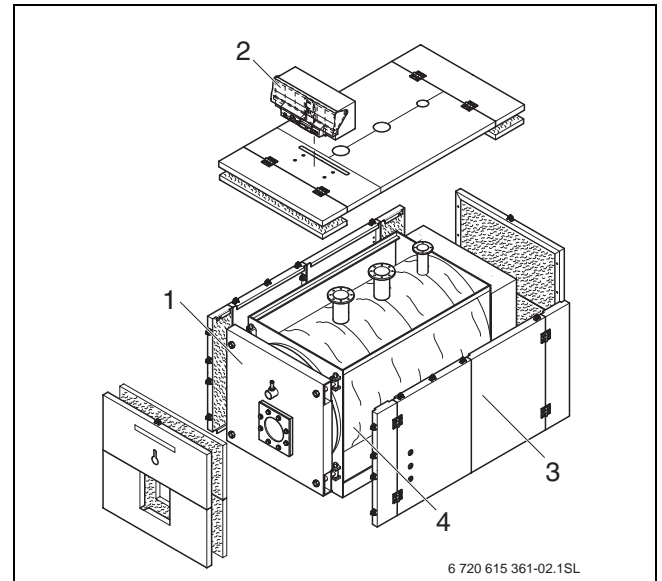
Рис. 1 Специальный отопительный котел Logano SK645 / SK745, работающий на дизельном/газовом топливе
