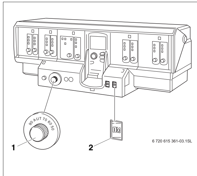
Рис. 2 Система управления (например: Logamatic 4311)
