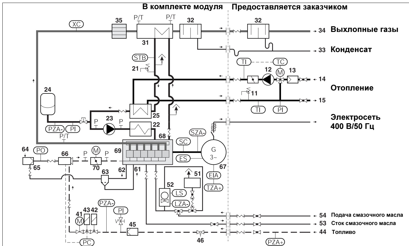
Рис. 2 Устройства контроля
