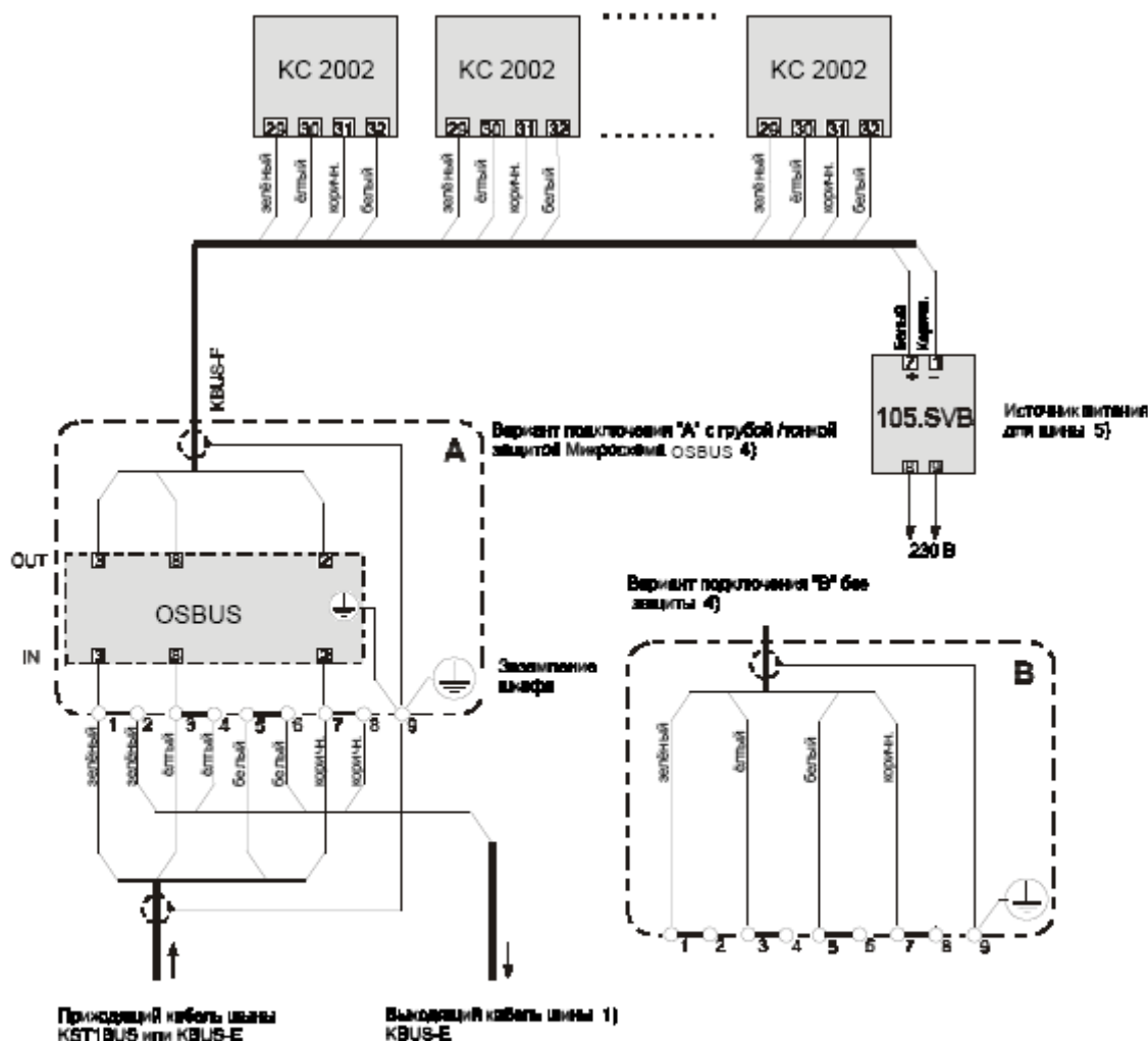
Рис. 4-12 Схема подключения в одном шкафу нескольких KC 2002
