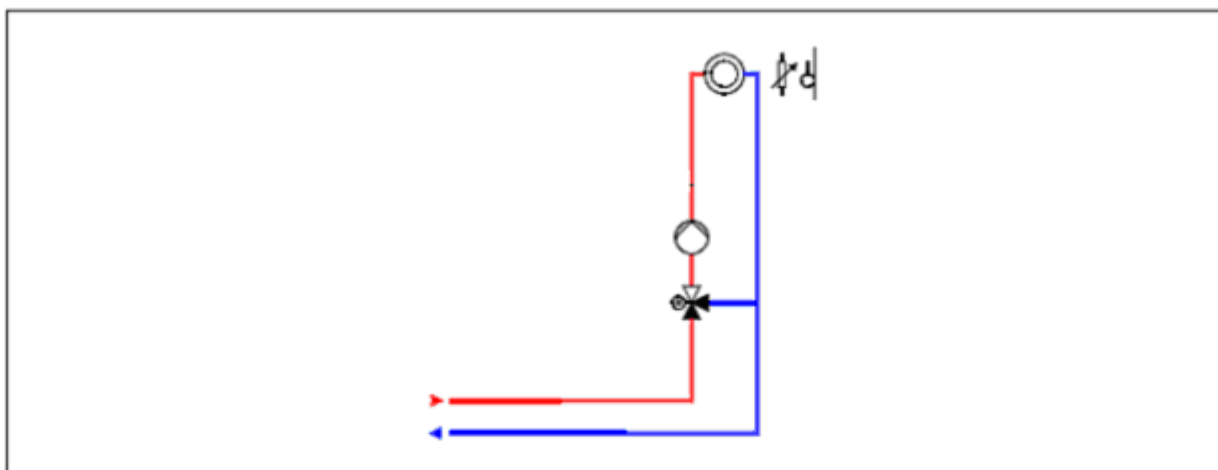
Схема 14: смешанный контур отопления (управляемый температурой помещения с дистанционным управлением помещения)
