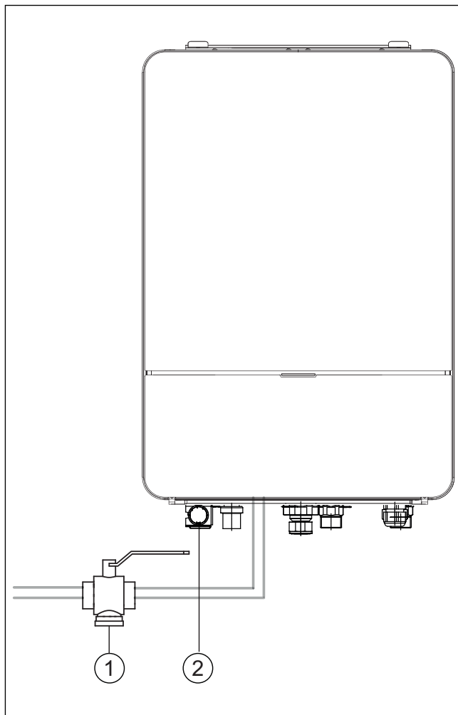
Рис. 7 Внутренний блок AWB
