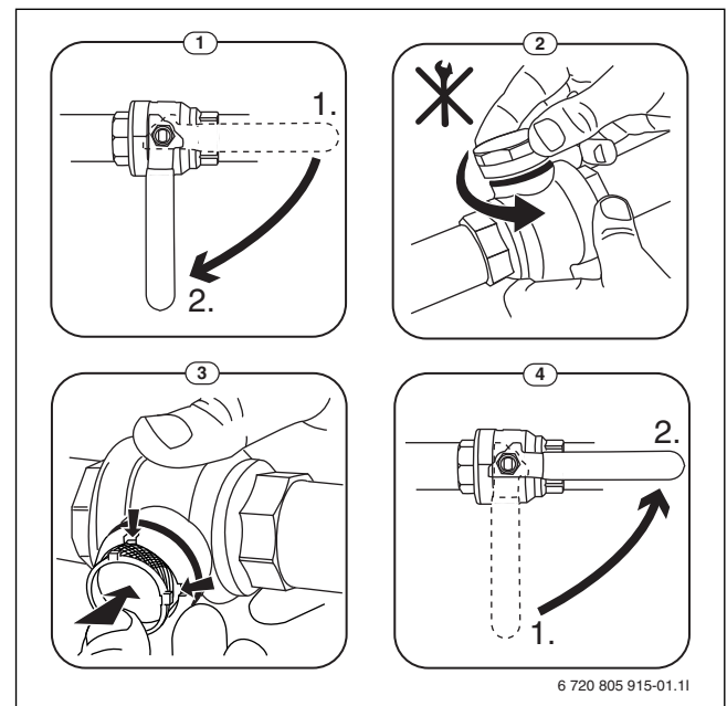
Рис. 8 Чистка сетчатого фильтра
