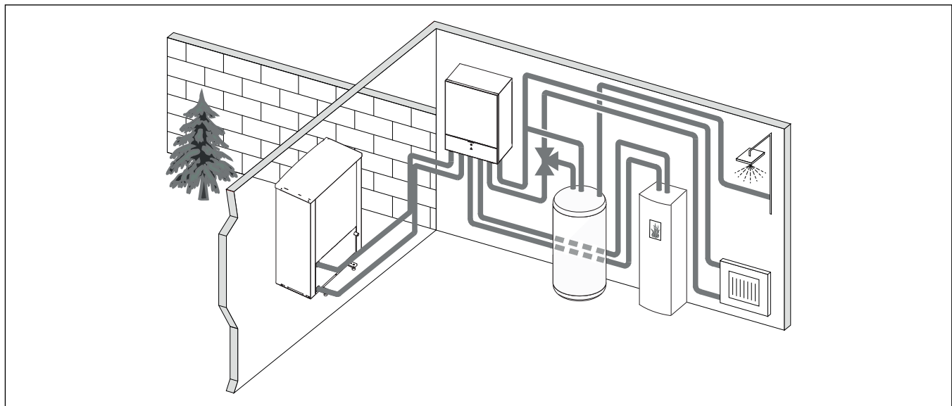
Рис. 3 Тепловой насос Compress 7000i AW, внутренний блок AWB со смесителем, внешний бак-водонагреватель и отдельный дополнительный нагреватель
