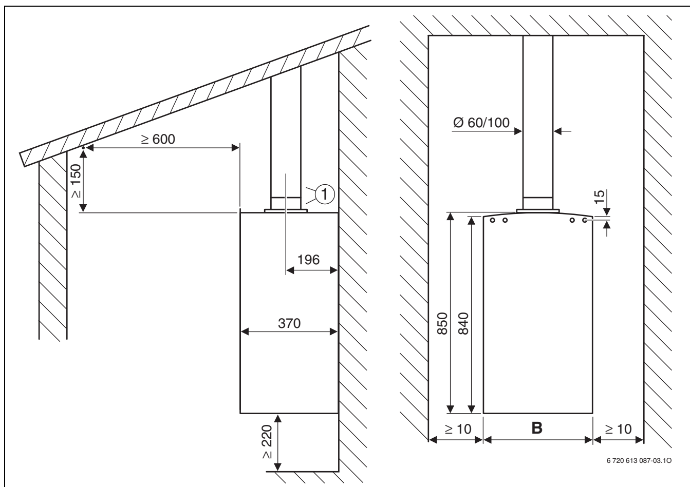
Рис 6 Наклонная крыша
