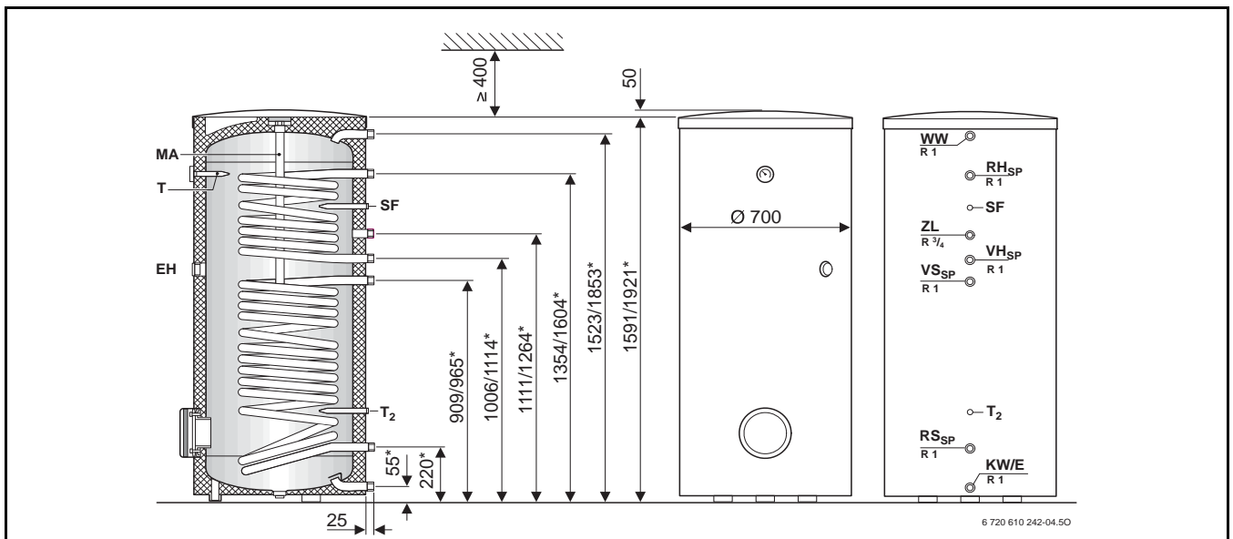
Рис 2 Размеры после косой черты относятся к следующему большему исполнению бойлера.
