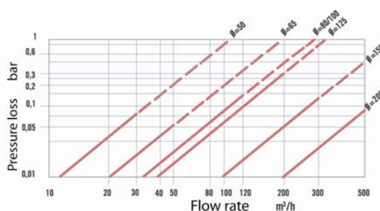
Диаграмма потери давления
