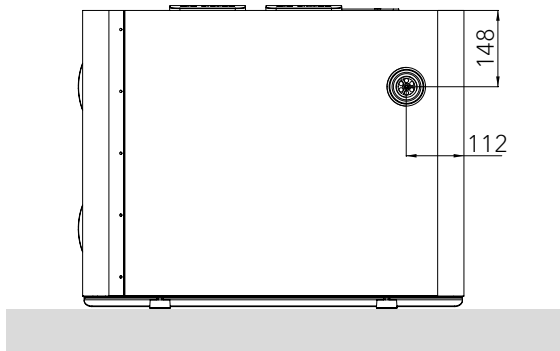
Вид снизу
