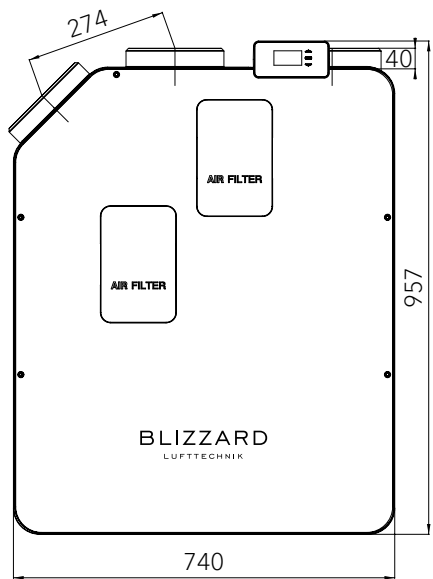
Вид спереди
