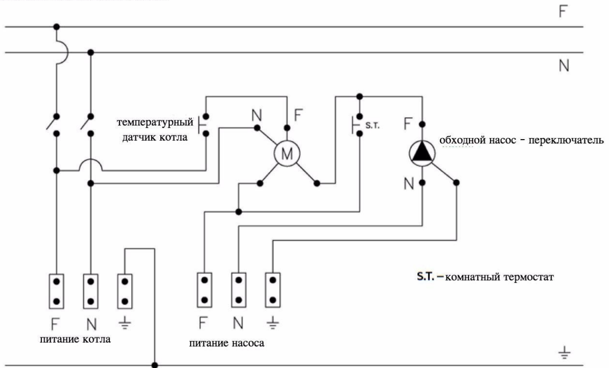
Электрическая схема 2
