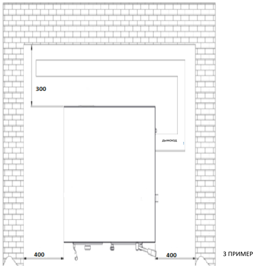
Рис. 1: Минимальное расстояние между котлом и стенами котельной
