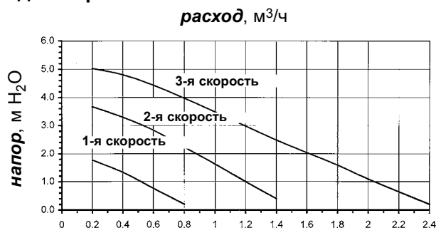
Рис. 12. Кривые расход/напор
