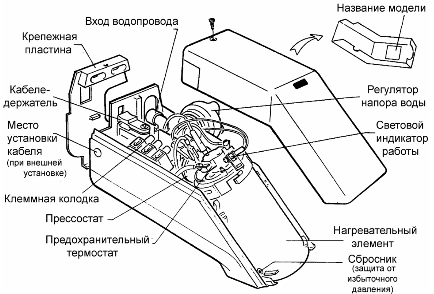
Рис. 1.0 Устройство водонагревателя
