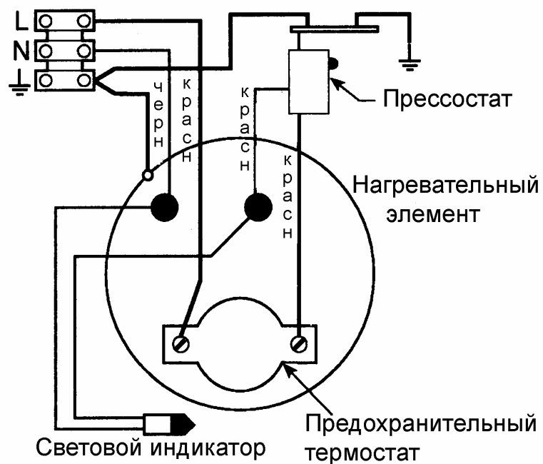
Рис. 1.1 Схема подсоединений
