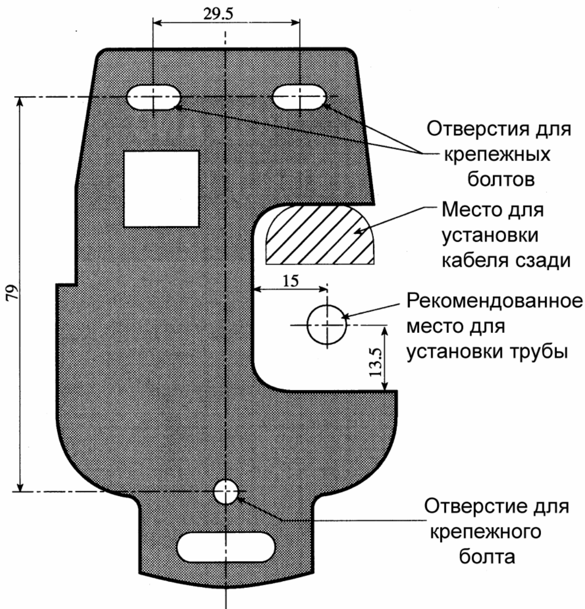
Рис. 4.5 Фиксация крепежной пластины на стене и подсоединение к системам
