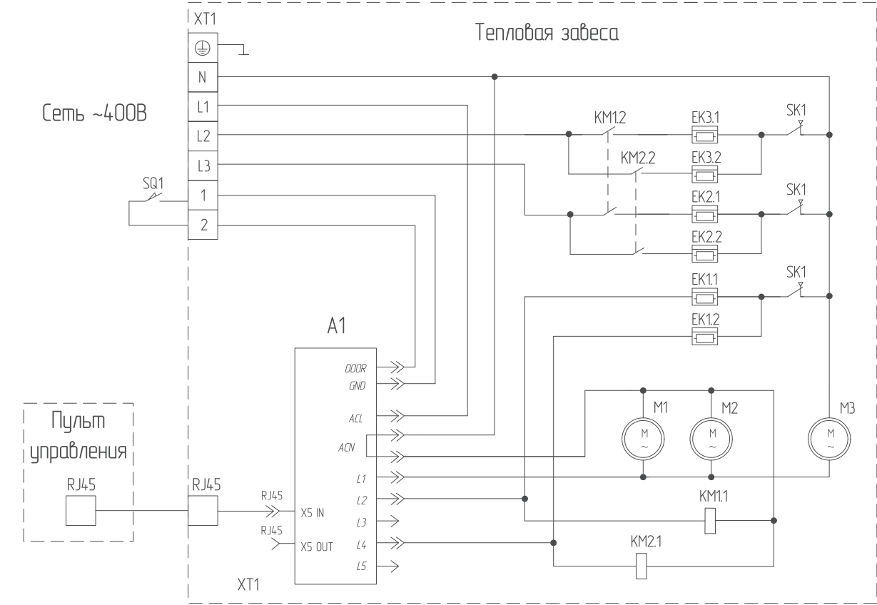
Подключение ВНС-L15-S09 (-М) к пульту ВНС-S
