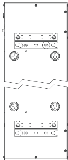
Схема крепления занавес серии PS вертикально к стене с помощью кронштейнов
