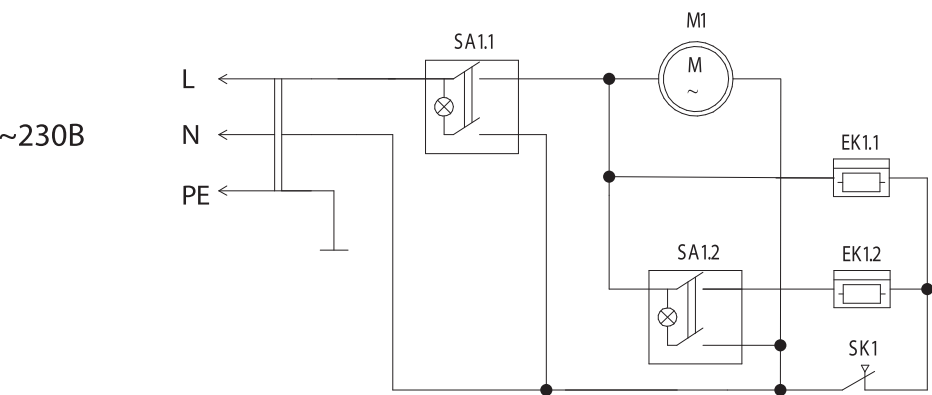
Подключение ВНС-СЕ-3 и ВНС-СЕ-3Л
