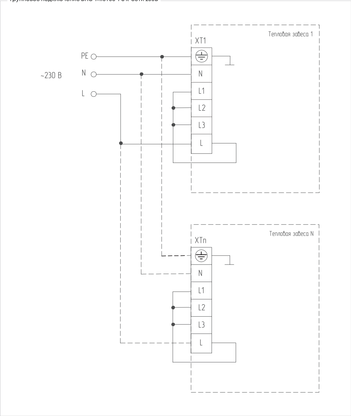
Групповое подключение ВНС-М10Т06-PS к сети 230В
