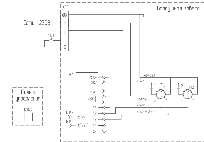
Подключение завес ULTRA без нагрева к пульту BRC-F
