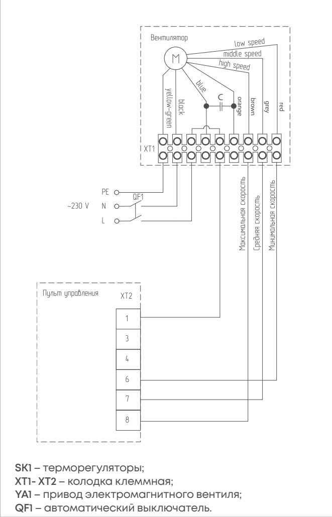
Подключение BDS-2-S к пульту BMC-1
