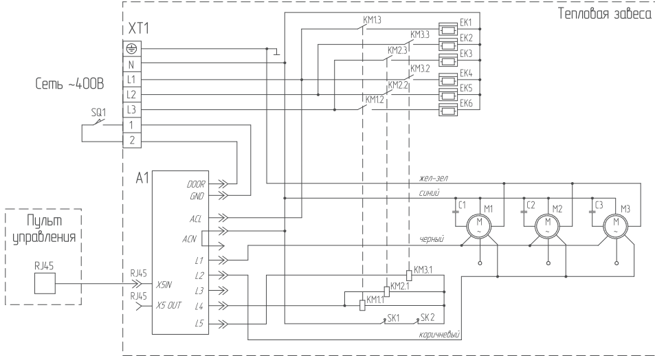
Подключение завес ULTRA с электрическим нагревом к пульту BRC-D1
