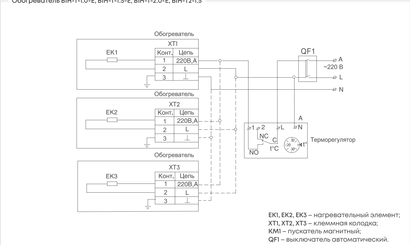
Обогреватель ВИН-T-1.0-Е, ВИН-T-1.5-Е, ВИН-T-2.0-Е, ВИН-T2-1.5
