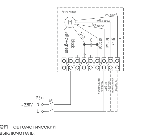
Подключение BDS-2-S к автоматическому выключателю
