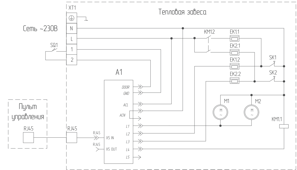
Подключение ВНС-L10-S06 (-М) к пульту ВНС-S
