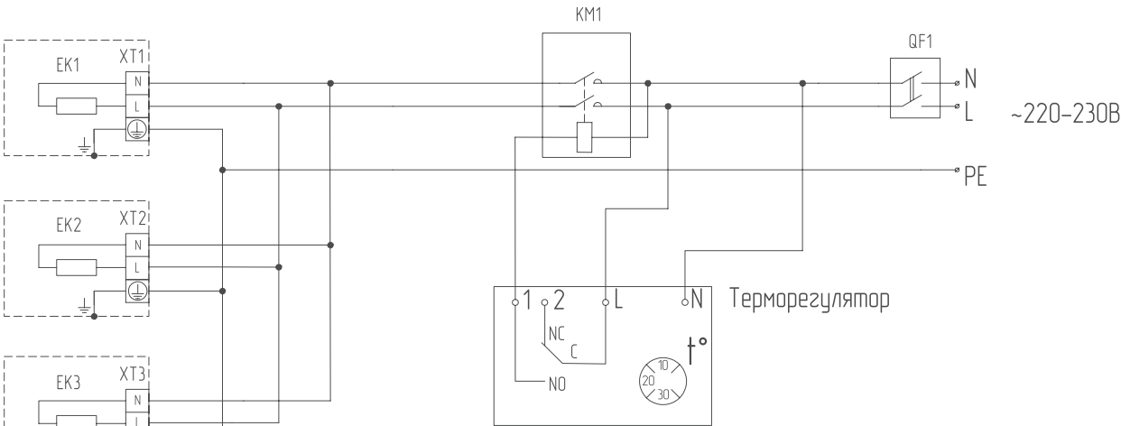
Обогреватель ВН-АПЛ-0.6-М; ВН-АПЛ-0.80-М; ВН-АПЛ-1.0-М, ВН-АПЛ-1.5-М
