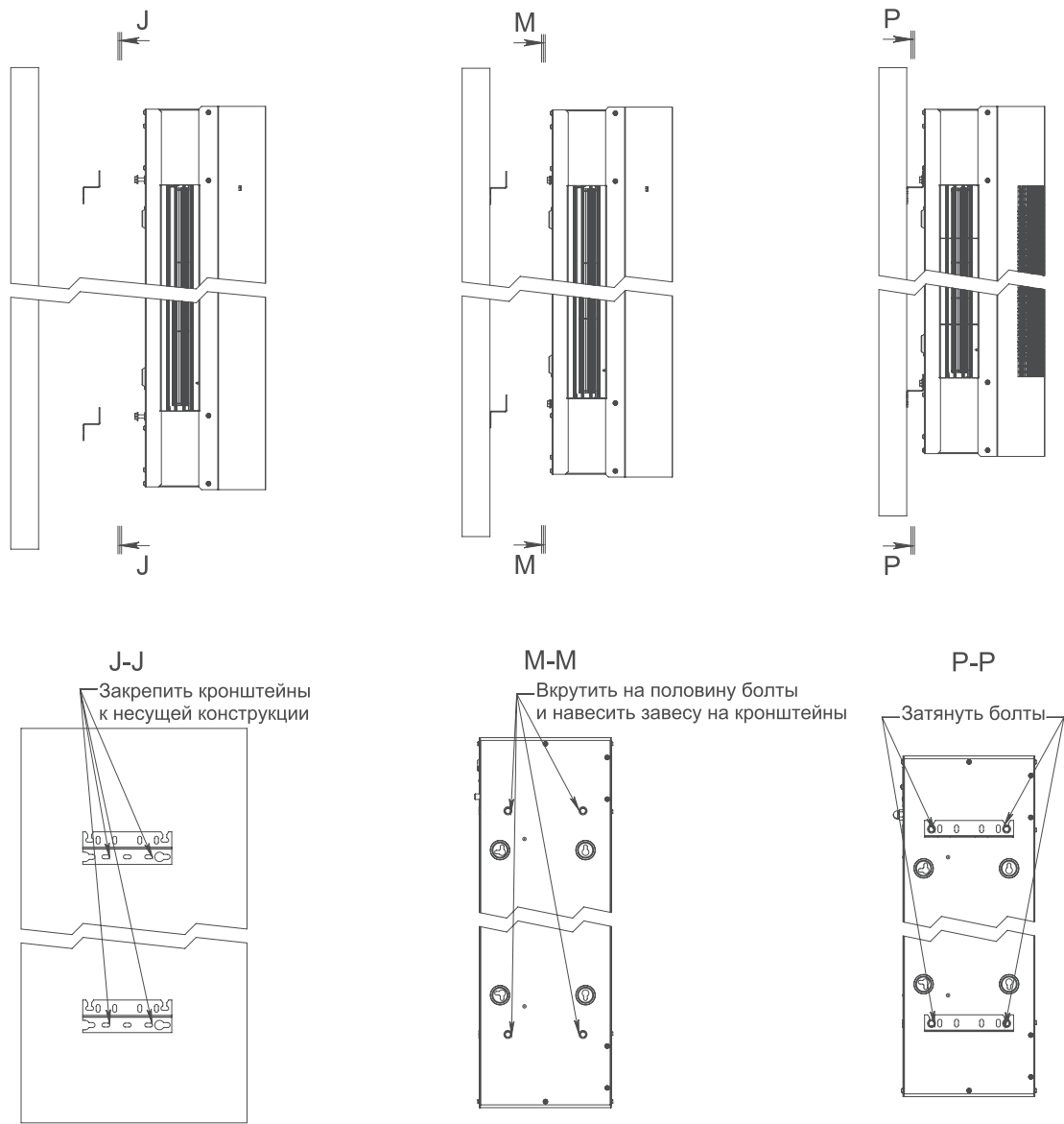
Схема крепления занавес серии PS вертикально к стене с помощью кронштейнов
