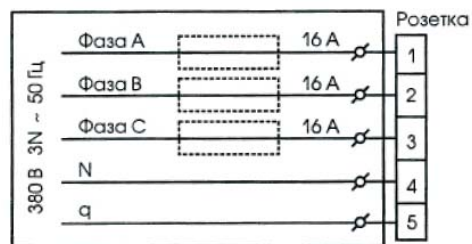
Рис. 2. Схема подключения розетки к стационарной электросети
