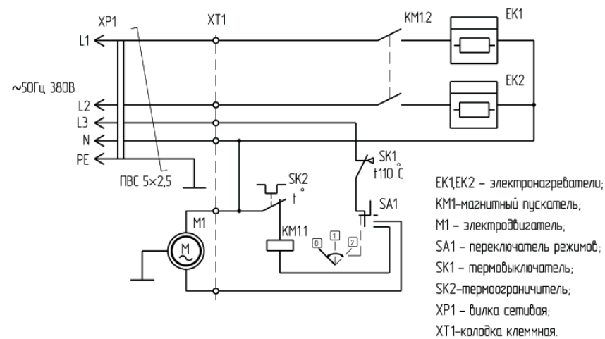
Рис.1. Схема электрическая
