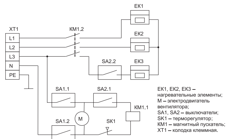
Рис. 1. Схема электрическая
