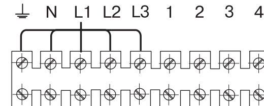
Рис. 5. Схема подключения ВНС-9 SR
