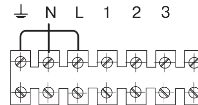
Рис. 4. Схема подключения ВНС-6 SR
