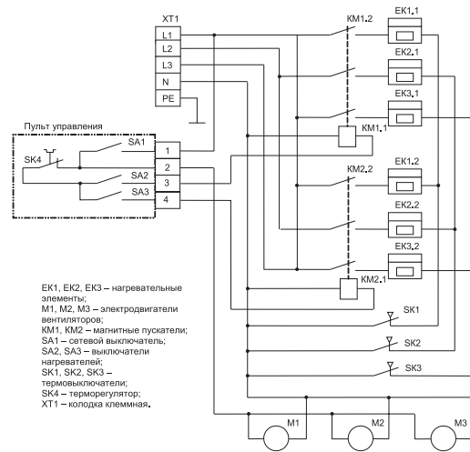
Рис. 3. Схема электрическая ВНС-9 SR
