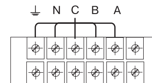
Рис. 4. Схема подключения
