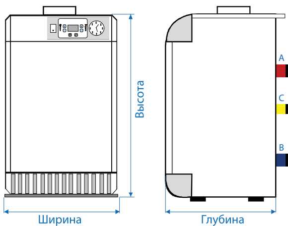
Рис. 4. Габаритные размеры.
