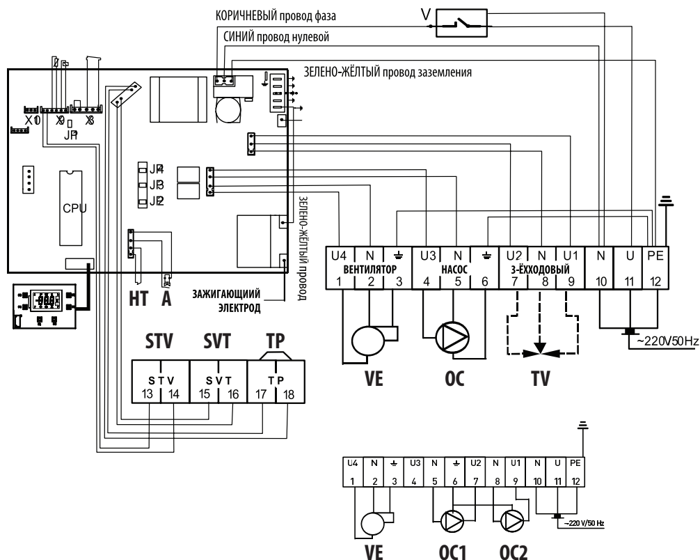
Рис. 6. Принципиальная электрическая схема.
