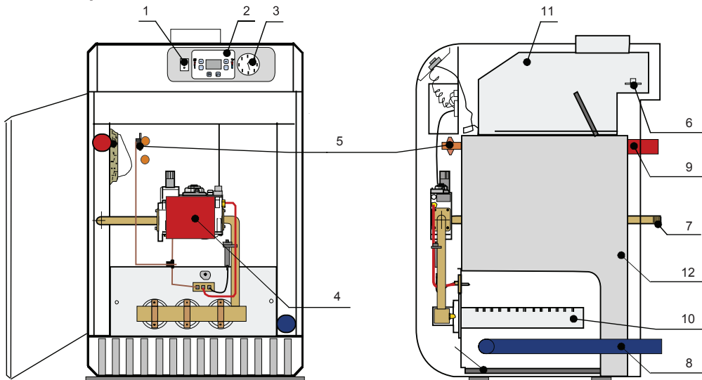
Рис. 1. Общий вид.
