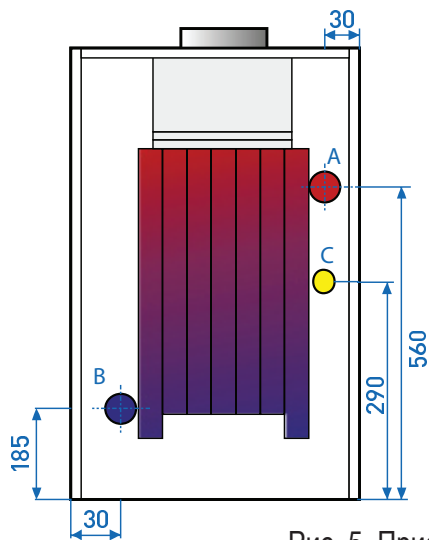
Рис. 5. Присоединительные размеры.
