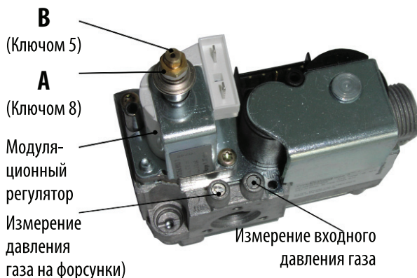
Рис. 6. Газовый клапан.
