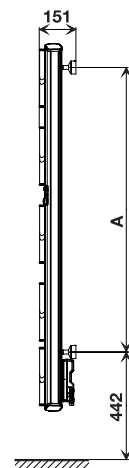
Вид сбоку
