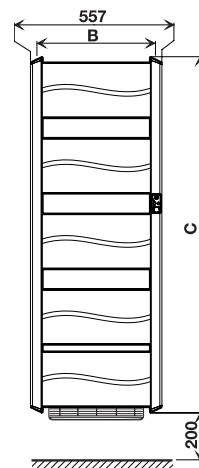
Вид спереди
