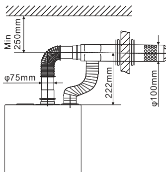
Коаксиальный дымоход из нерж. стали \varnothing 100/75 мм
