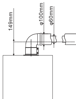
Коаксиальный алюминиевый дымоход \varnothing 100/60 мм
