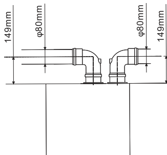
Раздельный алюминиевый дымоход \varnothing 80 мм
