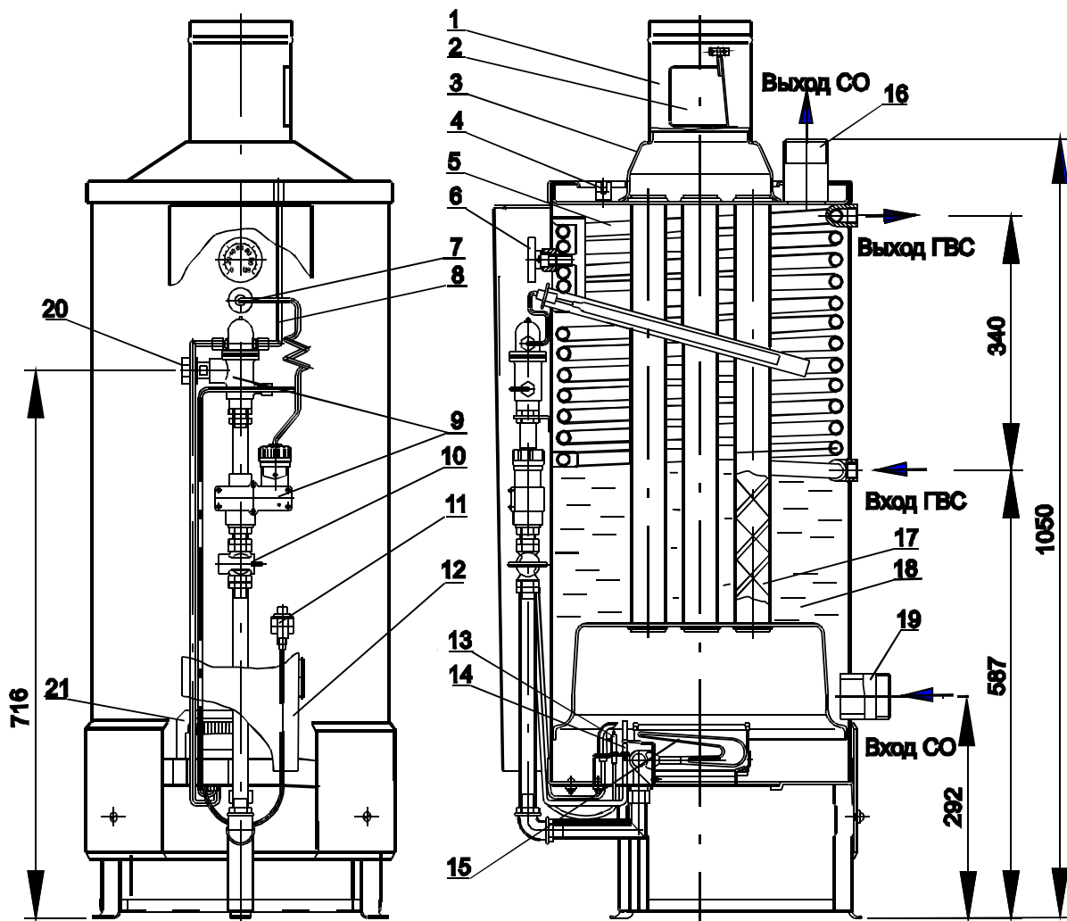
Рис.1 Аппарат комбинированный (отопительный) газовый бытовой Эконом
