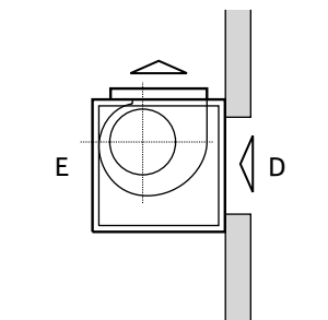
Компоновка VM9D
