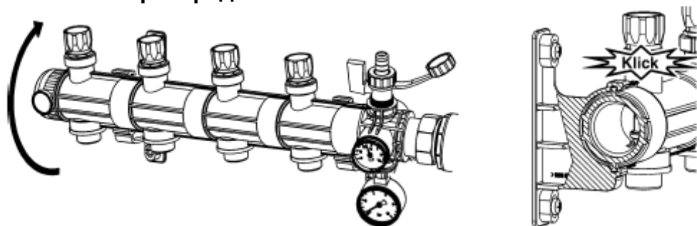
Рисунок 4: Монтаж распределителя
