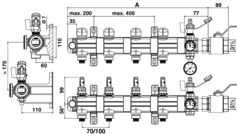
Рисунок 2: Габариты [мм], * при подключении G1 или G¾
