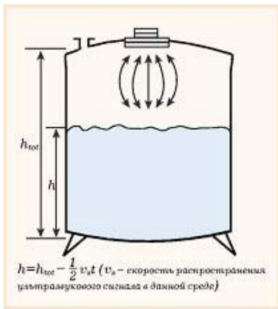
Рис. 24. Принцип реализации ультразвукового метода определения уровня
