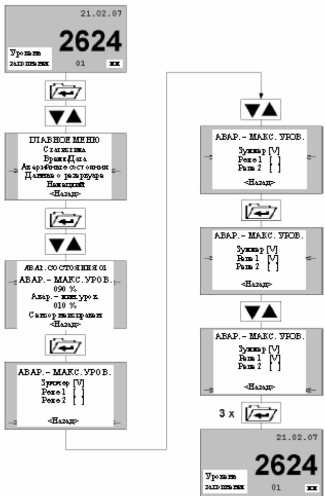
Рисунок 12: Регулировка зуммера/реле на примере максимального аварийного сигнала
