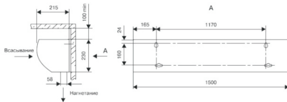
Рис. 1. Габаритные и установочные размеры
