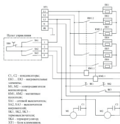
Рис 2. Схема электрическая
