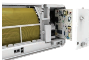
Кондиционер без функции I FEEL
