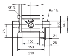
Резьбовое соединение (ВМН)
