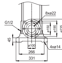
BMH(ч)64-6-2 ~ BMH(ч)64-8-1
