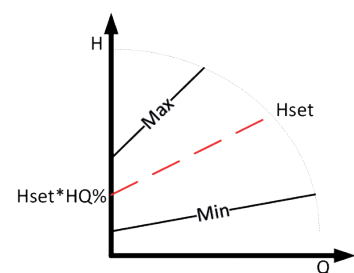
Пропорциональное давление
