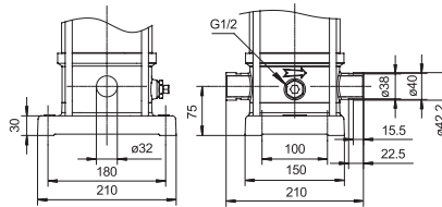
Соединение под хомут (ВМН)
