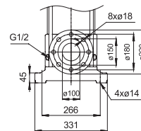
BMH(ч)64-1-1 ~ BMH(ч)64-5
