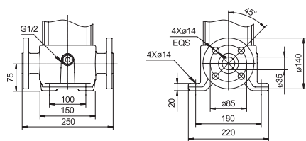
DIN фланец (ВМНч)
