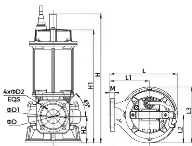
Однофазное исполнение
