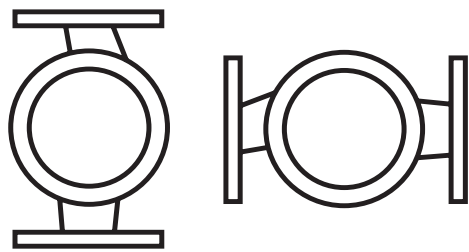
Правильная установка
