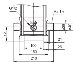
Резьбовое соединение (ВМН)
