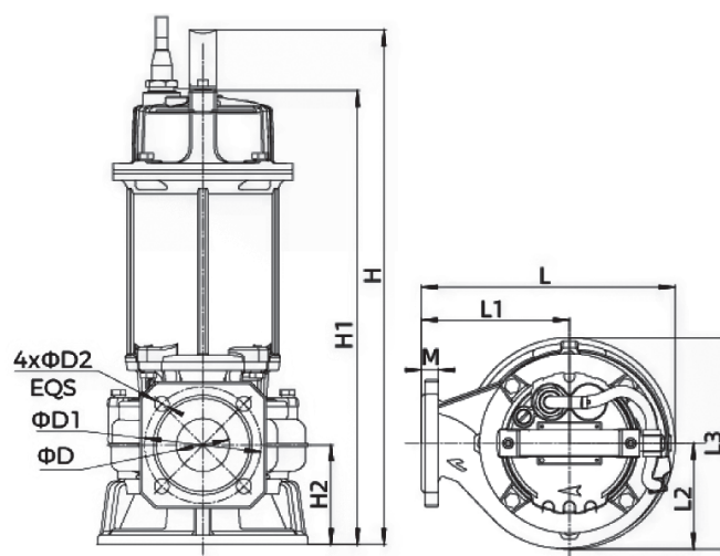
Трехфазное исполнение
