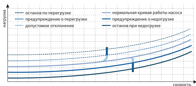
Рис. 4. Диаграмма нагрузки
