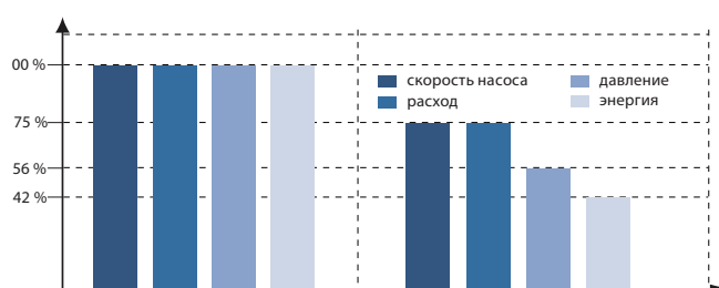
Рис. 5. Сравнительная диаграмма режимов работы насоса
