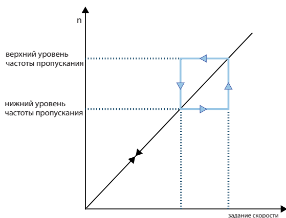
Рис. 2. Частота пропускания
