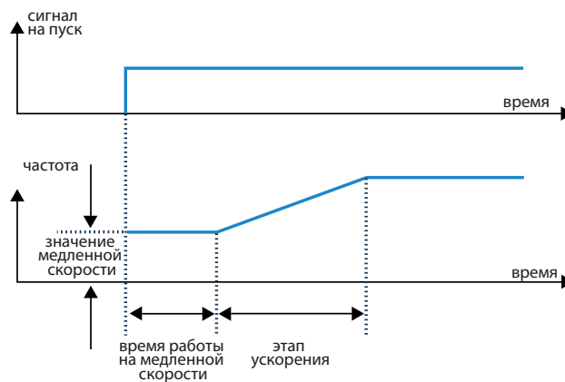
Рис. 3. Работа на медленной скорости
